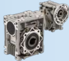
Doppelschneckengetriebe 0,06 - 1,85 kW i = 75 - 3000
